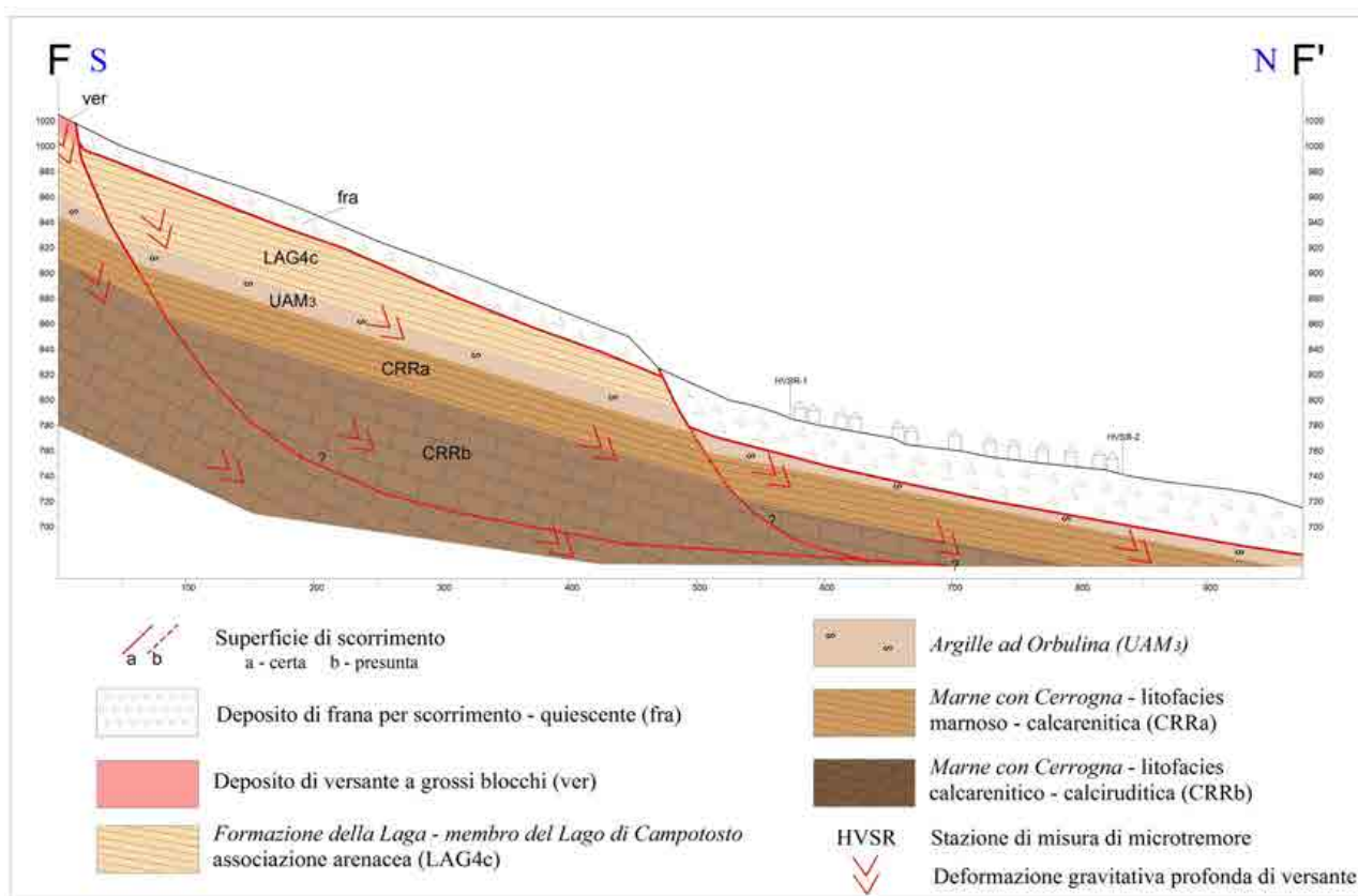
Fig. 13 - Sezione geologico-tecnica Caparrecce - abitato di Intermesoli.
